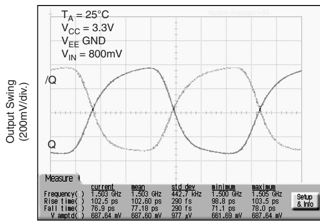
1.5GHz Output
