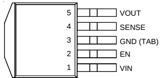
TO-263-5 RT9172S-□□xM5
