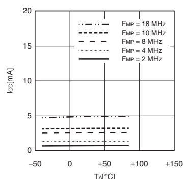
I_{CCS} - T_A
