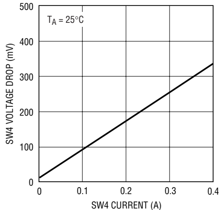
SW4 V_{\text{CESAT}}
