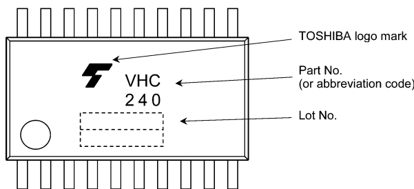
74VHC240FT
