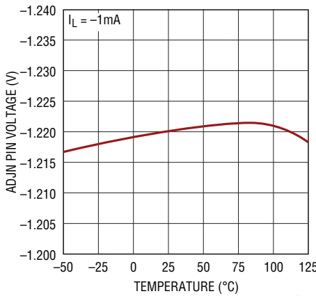
LT3032 ADJN Pin Voltage
