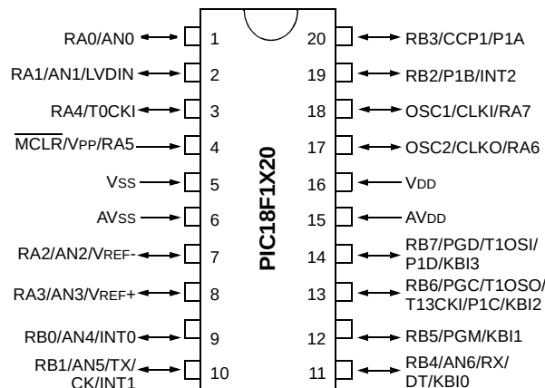
20-Pin SSOP
