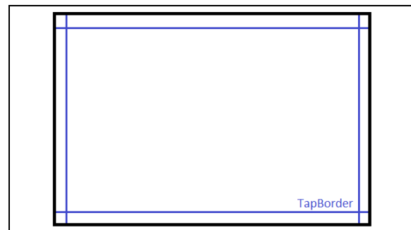
FIGURE 11-4: TAPBOARDER PARAMETER
