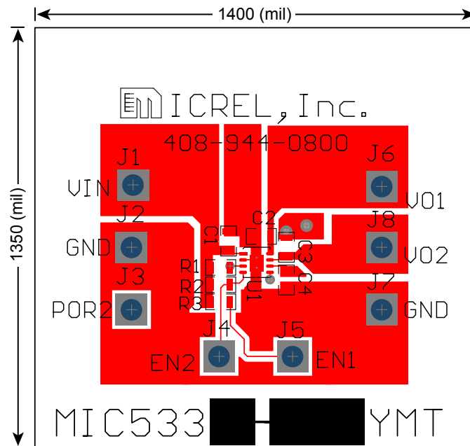
Top Layer
