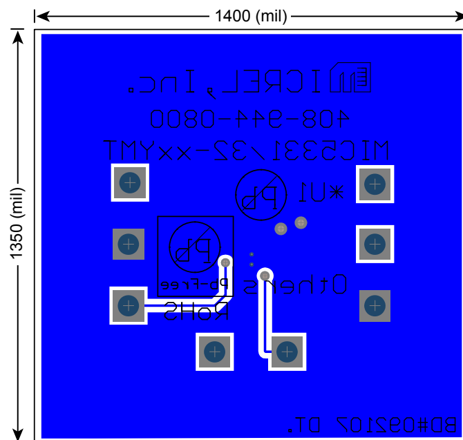
Bottom Layer
