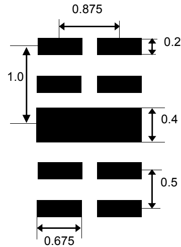
Package : DFN2510P10E
