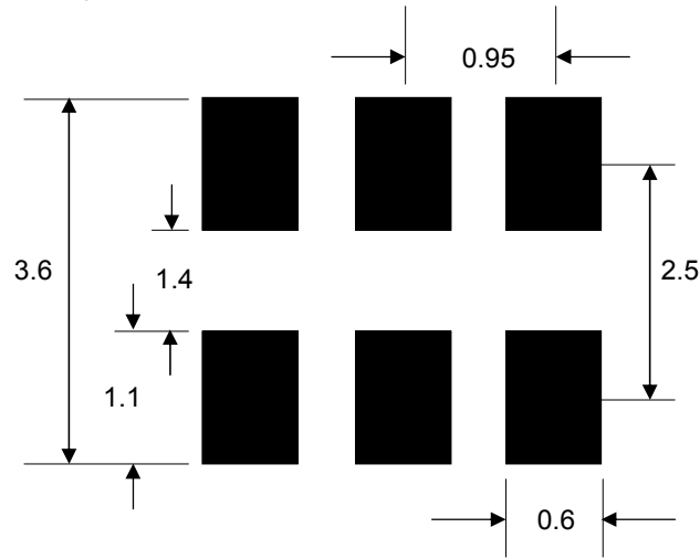
Package : SOT23-6L
