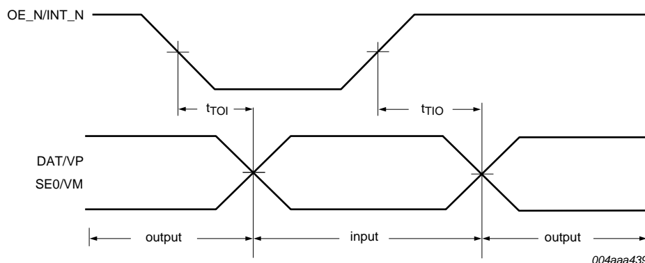
Fig 20. SIE interface bus turnaround timing
