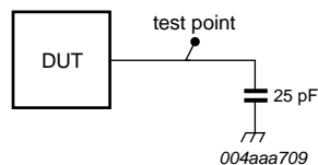
Fig 23. Load on pins VM, SE0/VM, VP, DAT/VP and RCV
