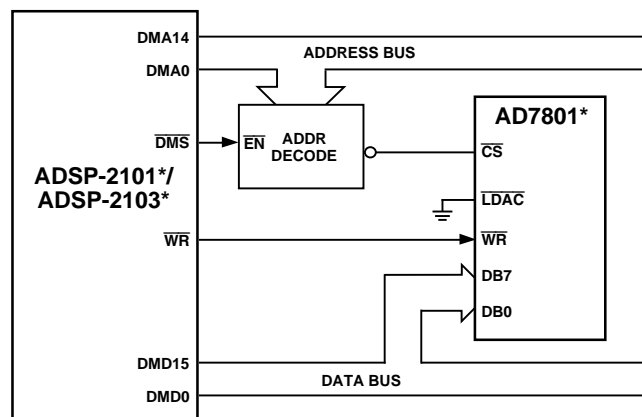
Figure 29. AD7801-ADSP-2101/ADSP-2103 Interface
