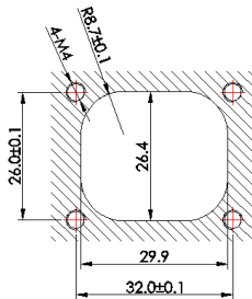
面板安装孔尺寸 Panel Size
