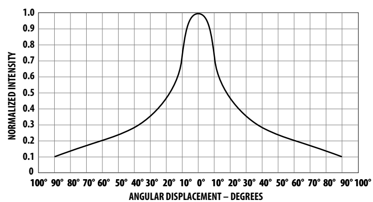
Figure 9: HLMP-Q102/-Q152
