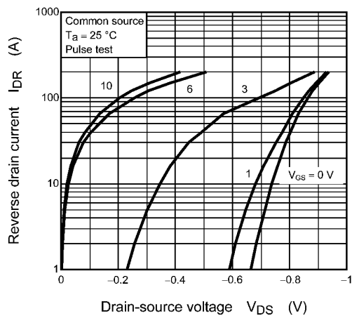
Fig. 9.7 I_{DR} - V_{DS}
