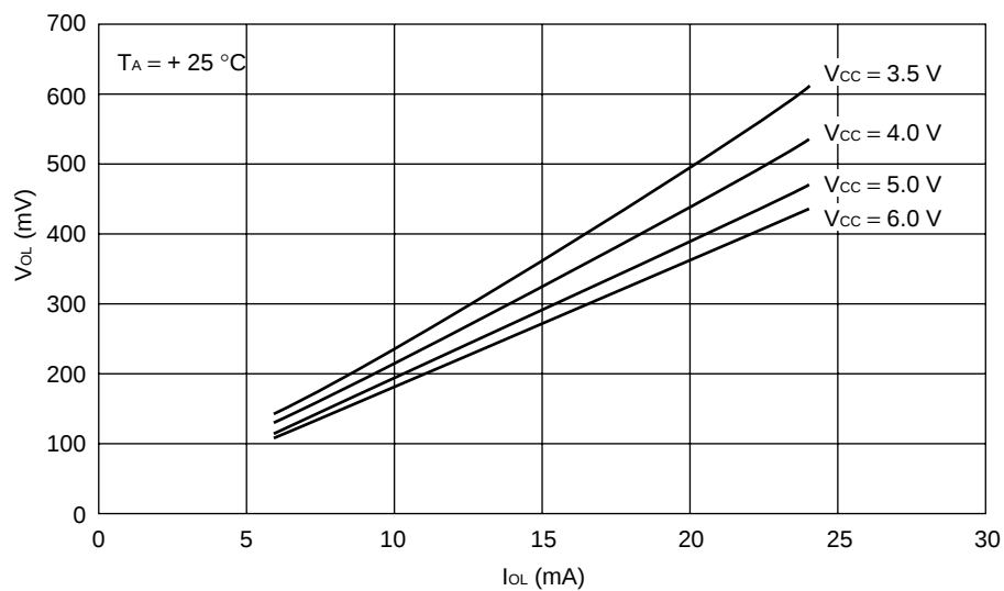
V_{OL} - I_{OL} P20 to P27
