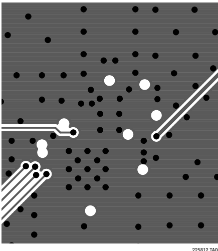
Inner Layer 3
