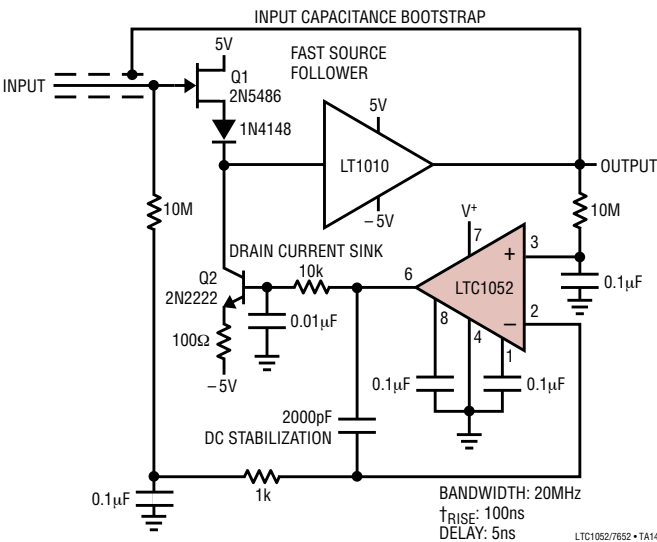
LTC1052/7652 • TA14
