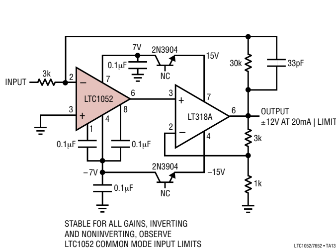
LTC1052/7652 • TA13
