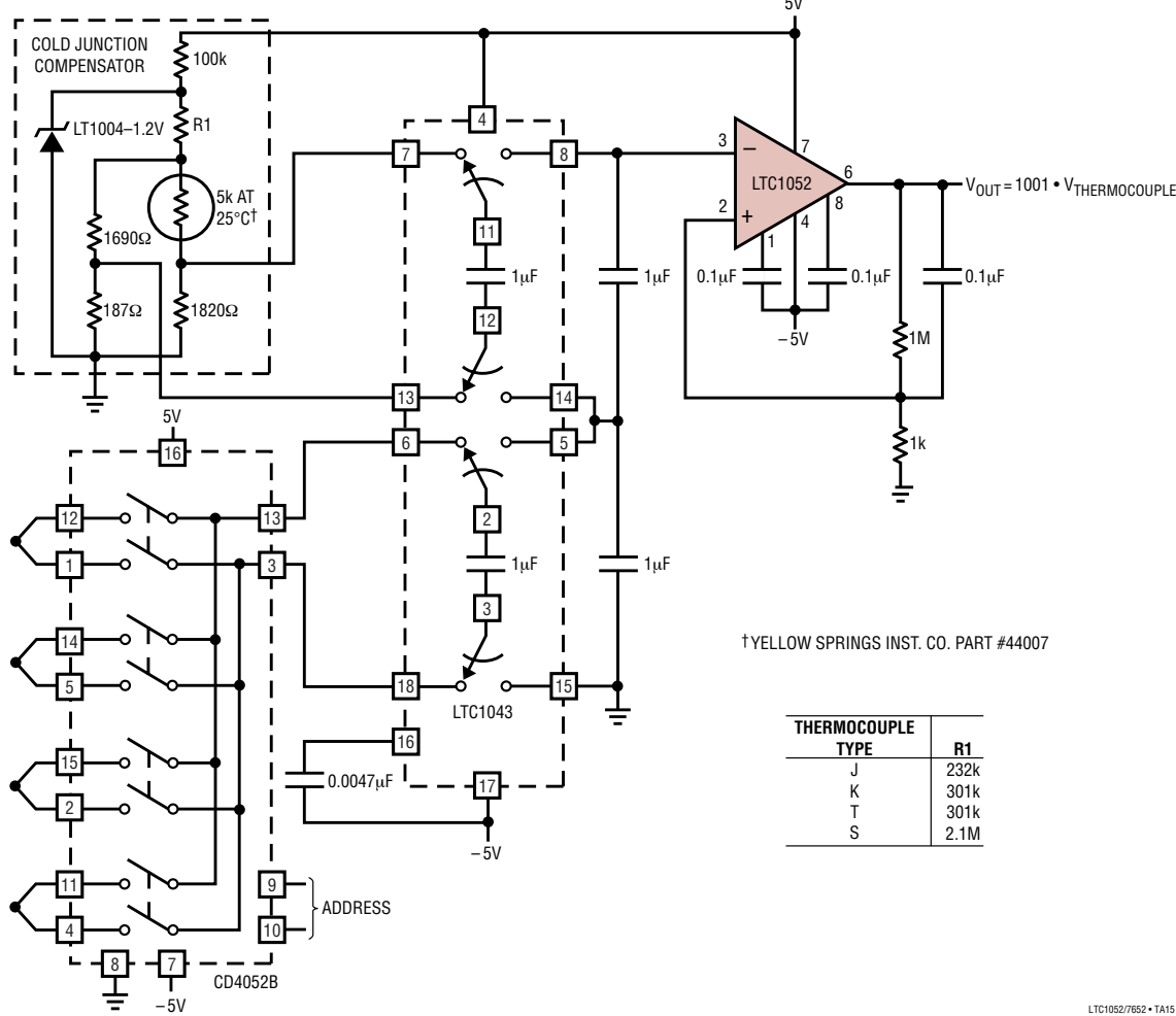
LTC1052/7652 • TA15
