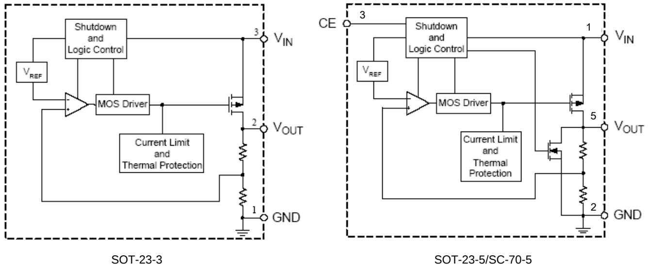
SOT-23-3
