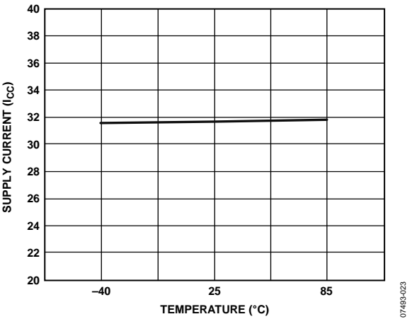
Figure 18. Supply Current ( I_{CC} ) vs. Temperature with ALS Asserted, I_{BIAS} = 11\text{ mA}
