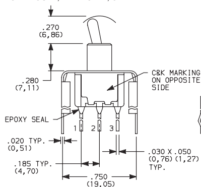
7101MD9_BE SPDT
