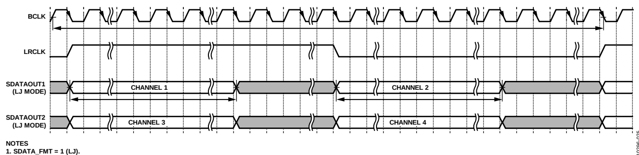
Figure 25. LJ Audio Format
