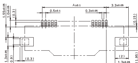
基板取付寸法 MOUNTING LAYOUT
