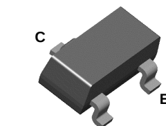
SOT-23 Mark: 1N
