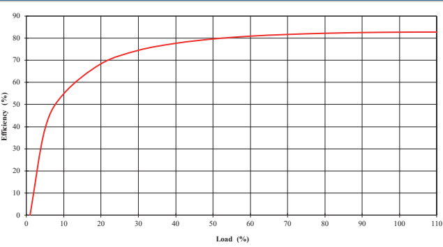
NMK0505TSAC
