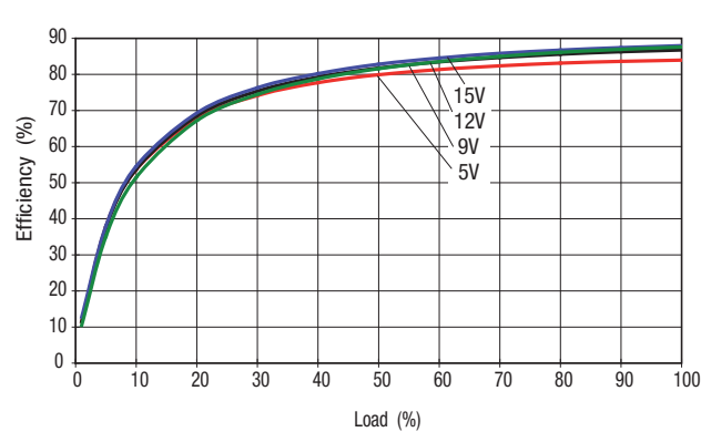
NMK05XXSC
