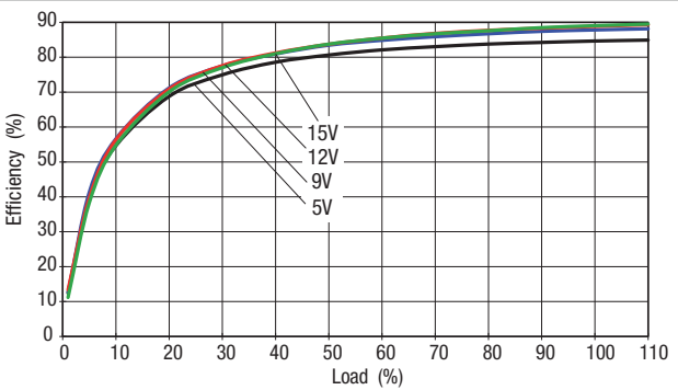
NMK24XXSC
