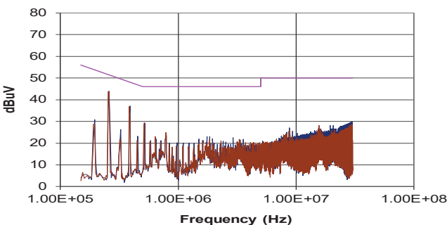
NMK0505TSAC (Average)
