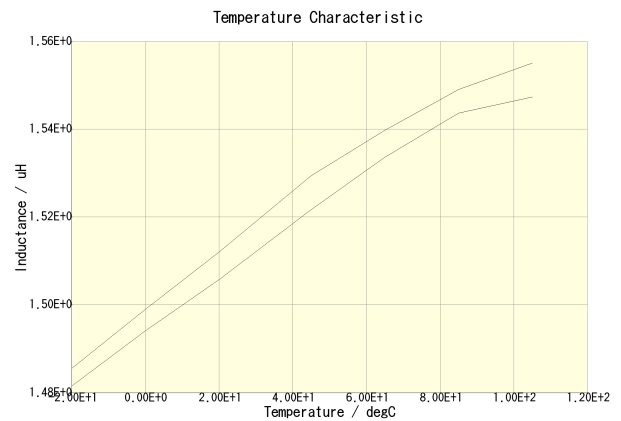
NLCV32T-1R5M-PF(DC = 0A)
