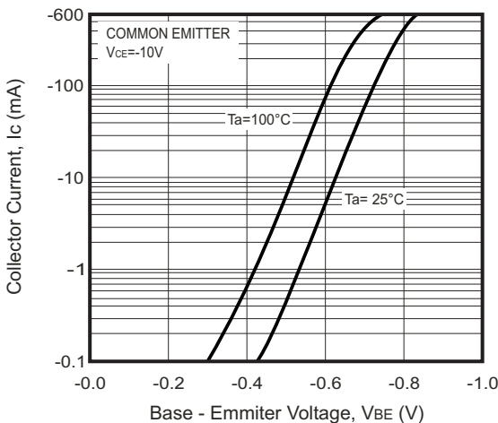
Fig.5 - I_c — V_{BE}
