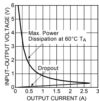
Si3445DV SOA
