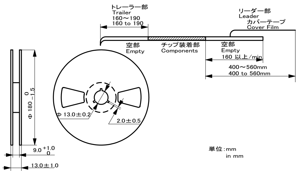
第4図 プラスチックリールの外形寸法図 Figure 4. Dimensions of Plastic Reel (CSTCW20M0X51-R0)
