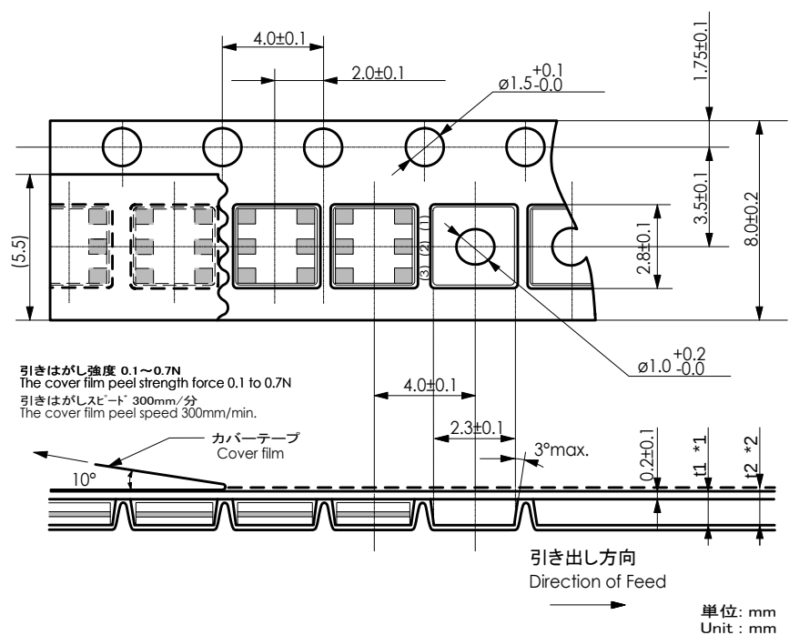
第3図 プラスチックテープの外形寸法図 Figure 3. Dimensions of Plastic Tape (CSTCW20M0X51-R0)
