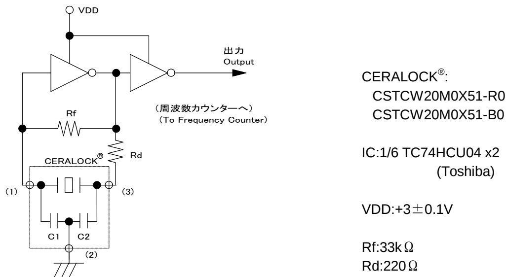
第2図 発振周波数測定回路 Figure 2. Test Circuit
