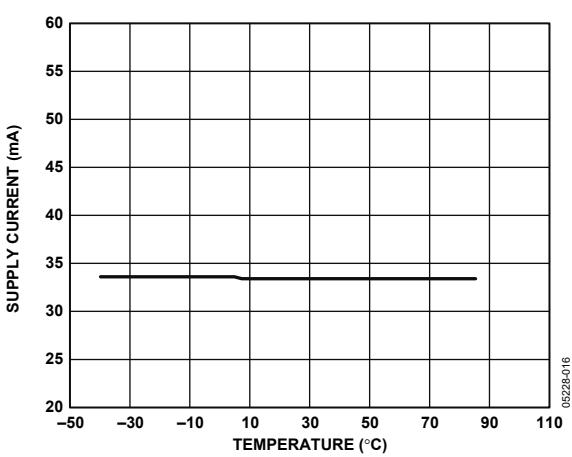
Figure 18. Supply Current ( I_{CC} ) vs. Temperature with ALS Asserted, I_{BIAS} = 20\text{mA}
