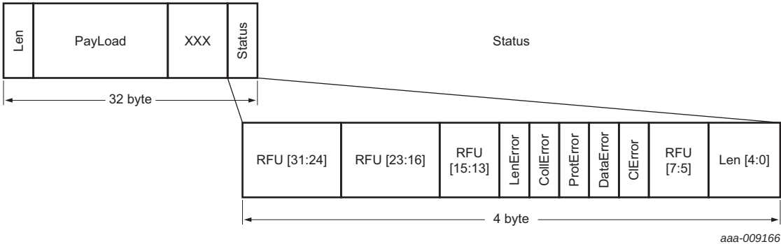
Fig 23. RxMultiple data format
