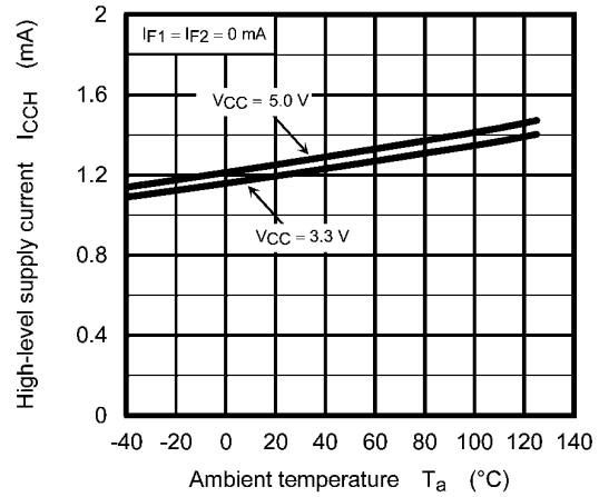
Fig. 12.2.8 I_{CCH} - T_a
