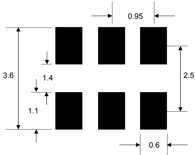
Package : SOT23-6L
