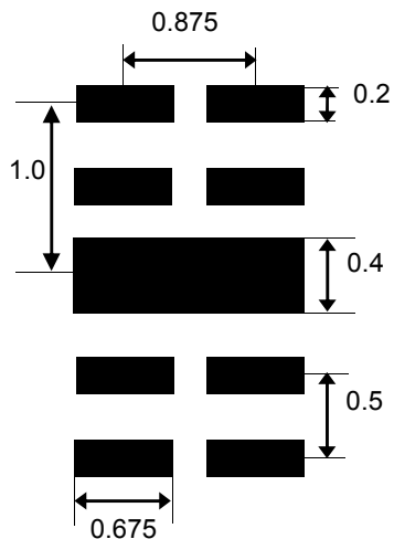
Package : DFN2510P10E
