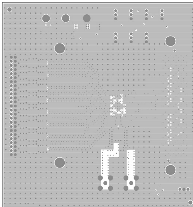
Inner Layer 2
