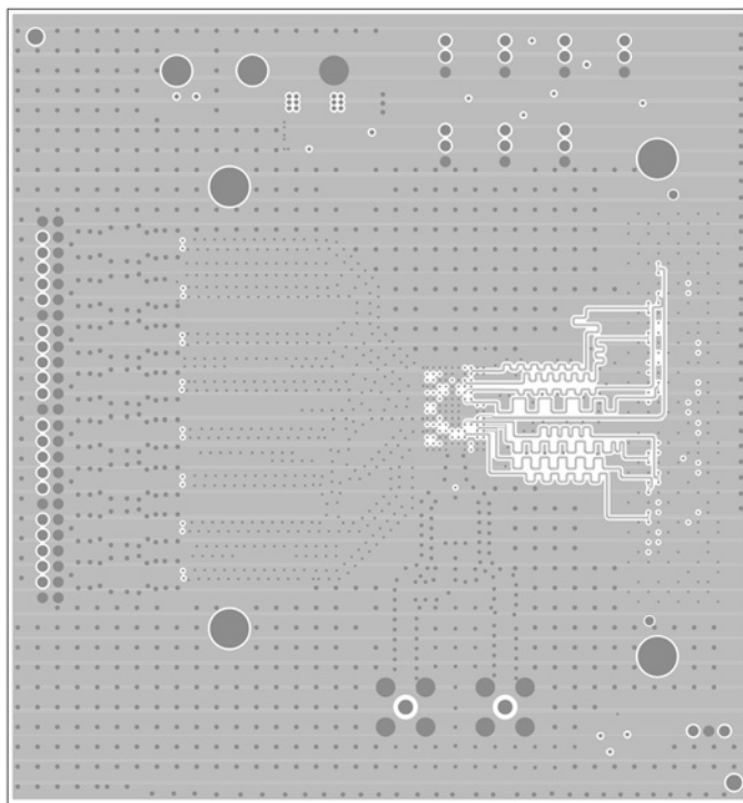
Inner Layer 5
