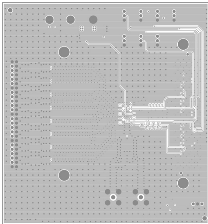
Inner Layer 4
