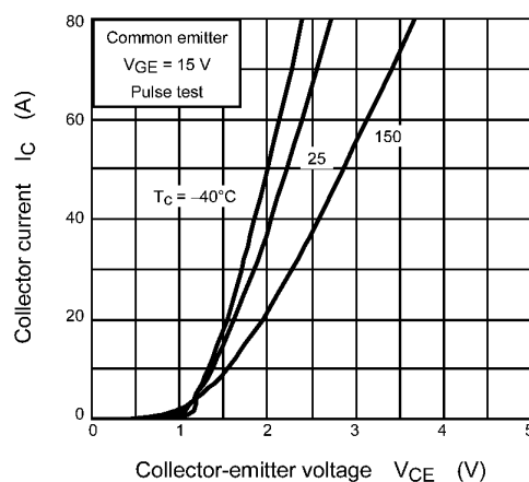
Fig. 8.4 I_C - V_{CE}
