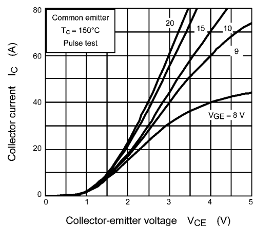
Fig. 8.3 I_C - V_{CE}
