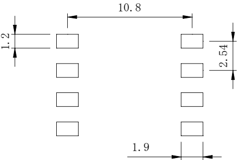
2-3. 推奨ランド寸法 (mm)
