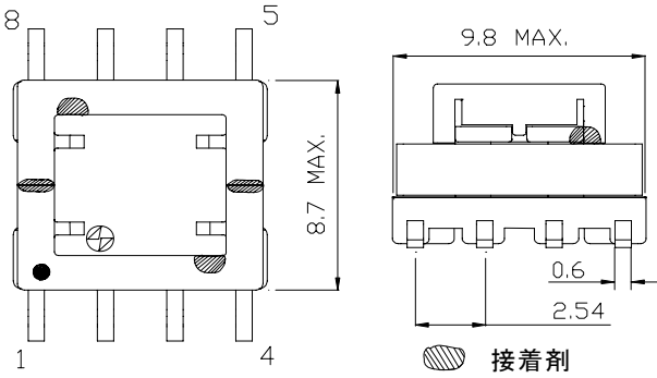
2-1. 寸法図 (mm) △3
