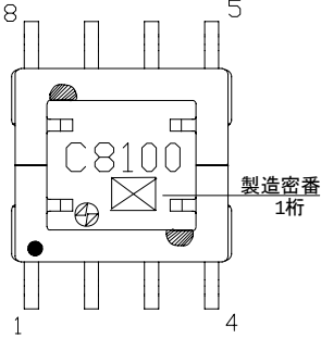
2-2. 捺印 △3
