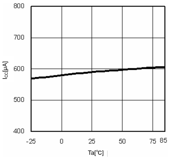
Fig.10 Ta-Icc
