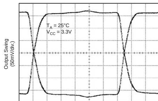
155MHz Output
