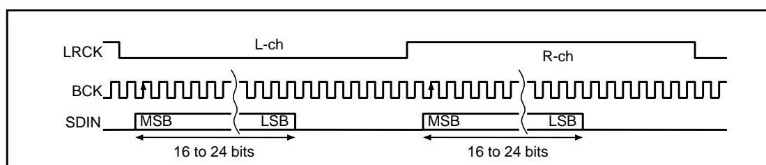
(1) : I²S data input
