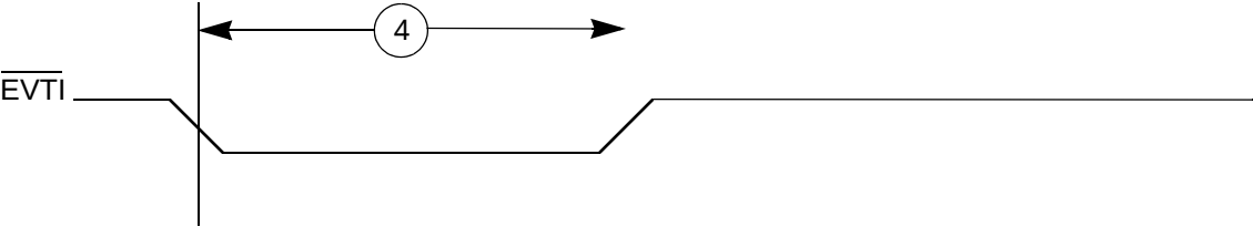
Figure 26. Nexus EVTI Input Pulse Width
