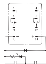
MY2N-D2
