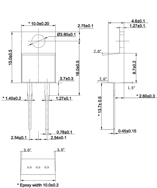
TO-220-AC
