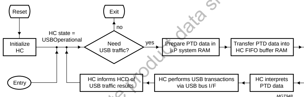
Fig 15. ISP1160/01 HC USB transaction loop.
