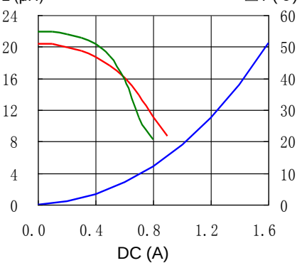
7. CDPH4D19FNP-220MC
