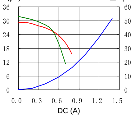
8. CDPH4D19FNP-330MC
