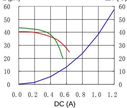
9. CDPH4D19FNP-470MC
