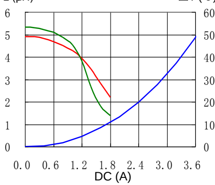
5. CDPH4D19FNP-100MC
