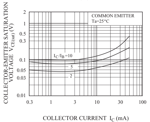
V_{CE(sat)} - I_C
