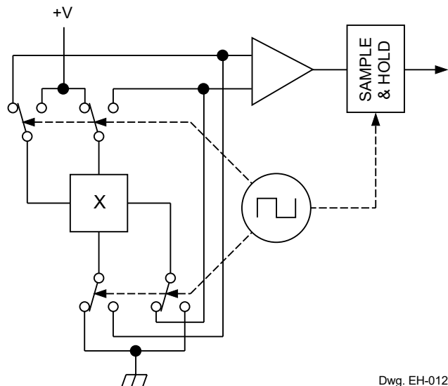
Dwg. EH-012-1
