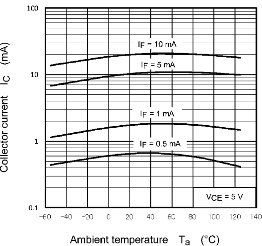
Fig. 11.12 I_C - T_a
