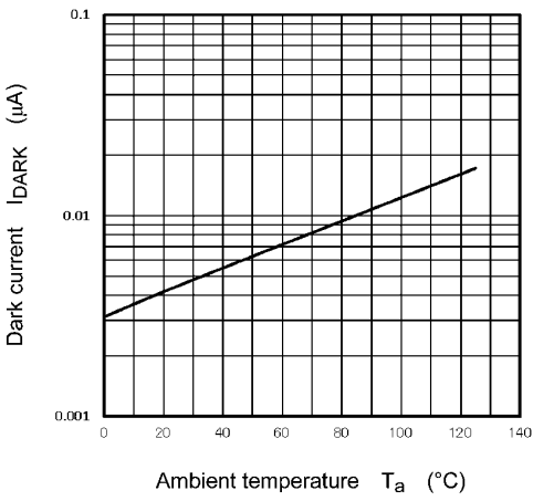
Fig. 11.10 I_{DARK} - T_a
