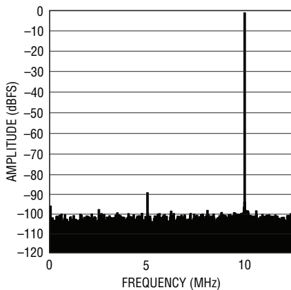
LTC2263-14: 8k Point FFT, f_{IN} = 140\text{MHz} , -1\text{dBFS} , 25\text{Mps}
