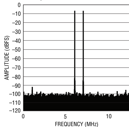
LTC2263-14: 8k Point 2-Tone FFT, f_{IN} = 68\text{MHz} , 69\text{MHz} , -1\text{dBFS} , 25\text{Mps}
