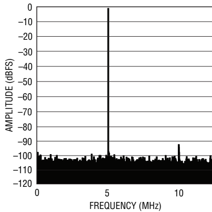
LTC2263-14: 8k Point FFT, f_{IN} = 5\text{MHz} , -1\text{dBFS} , 25\text{Mps}
