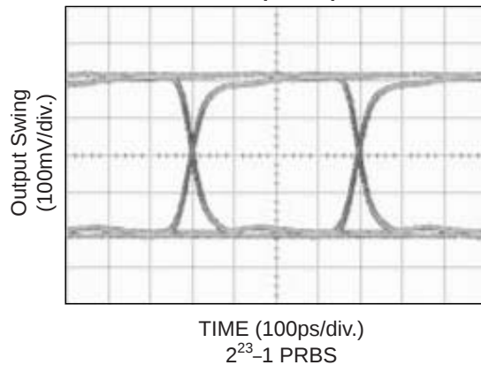
2.5Gbps Output
