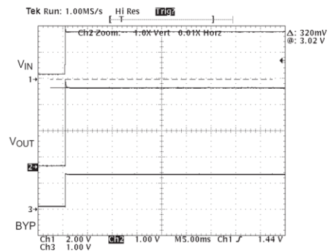
Fig. 15: Fast V_{IN} , No Load
